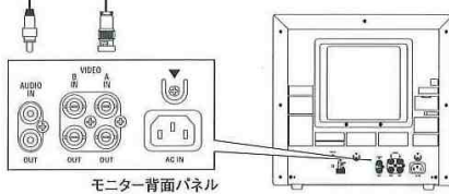
モニター背面パネル
